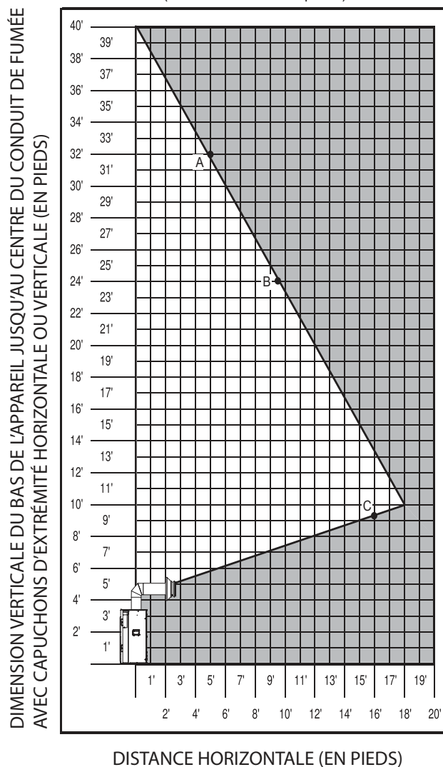
Graphique pour évacuation avec terminaison horizontale (Dimensions en pied)
