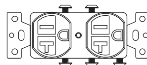
Prise électrique double 1x
