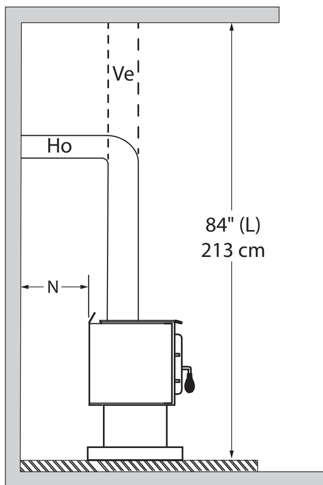
Figure 15: Développements - Côté
