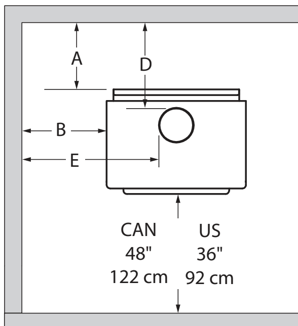
Figure 13: Développements - Dessus
